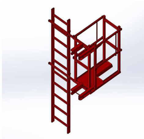
Schéma n°4 - Vue passerelle d'accès AMG cabine-mâtresse
